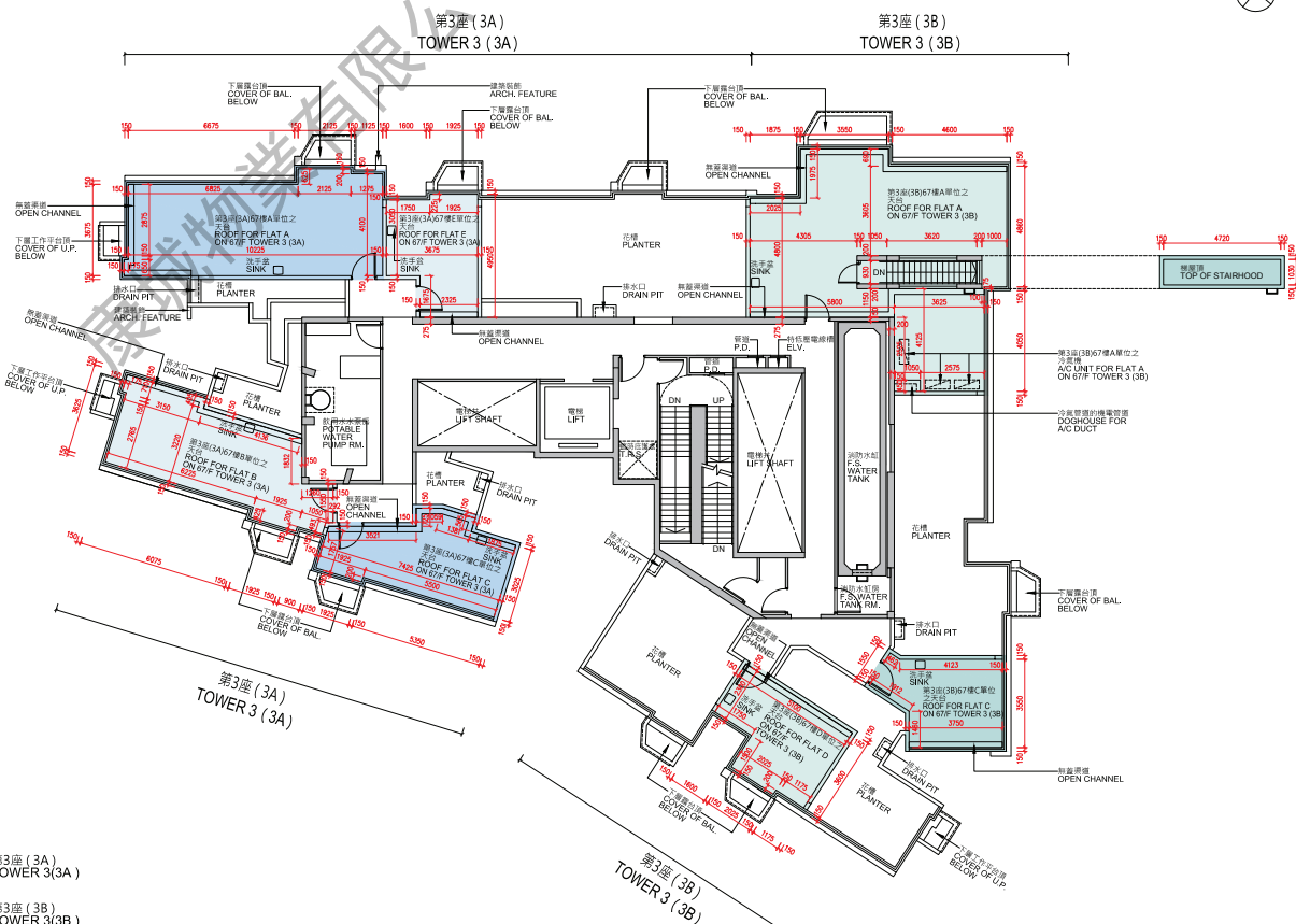
Tower 3 (3A & 3B) Roof Floor Plan 第3座(3A及3B)天台樓面平面圖
